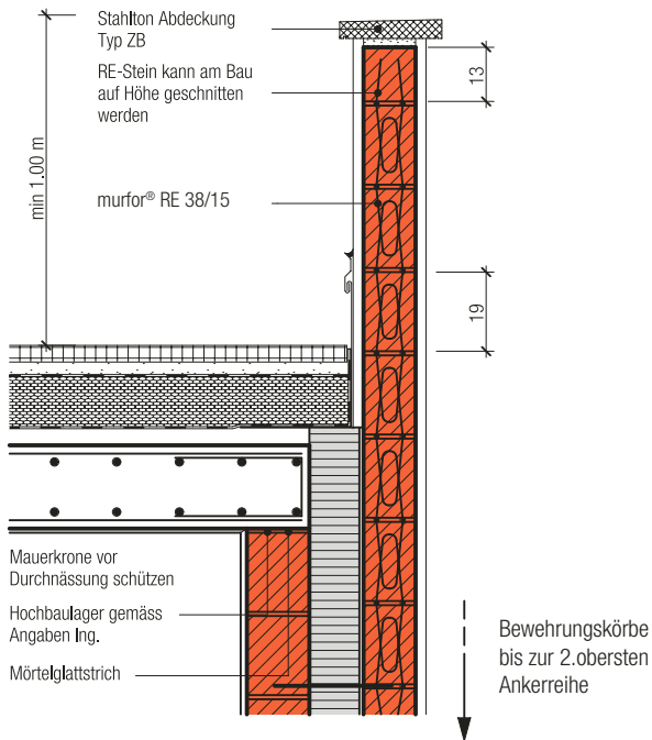
Auskragende Aussenschale
