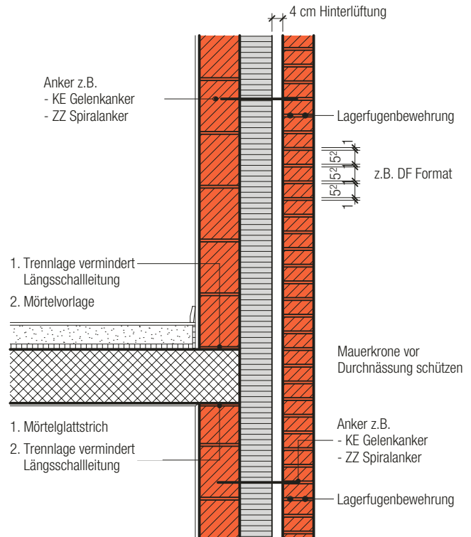
Schnitt A-A
