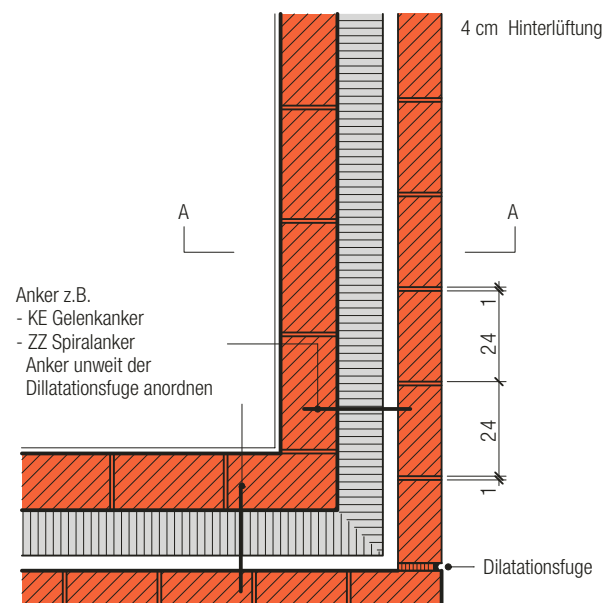
Grundriss Klinkersteinwand
