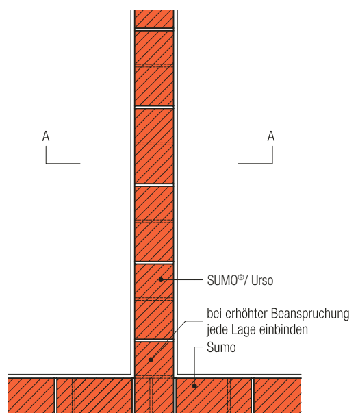
Grundriss Wände gleichzeitig gemauert 1. + 2. Schicht
