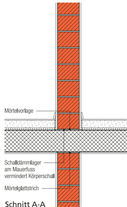
Schnitt A-A
