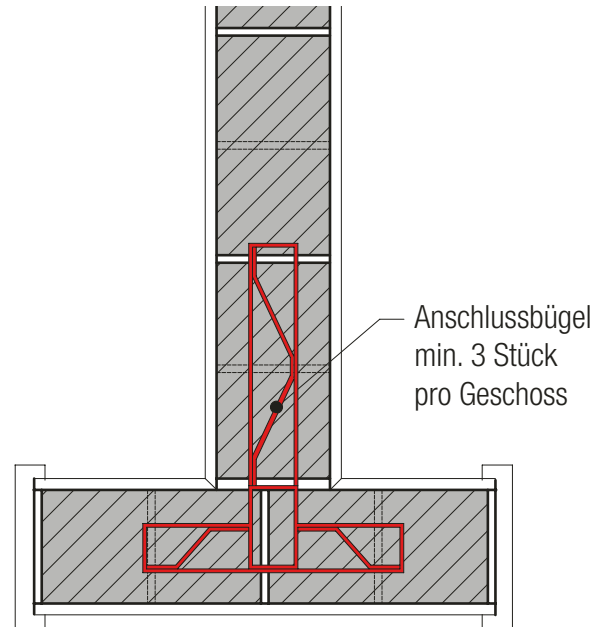
Anschlussbügel, Detail 2
