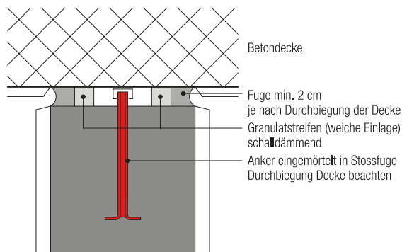
Schnitt
