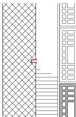
Metaldübel HKD-SR M6 setzen und mittels Einschlagwerkzeug spreizen
