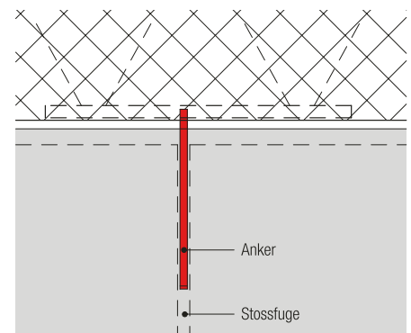
Ansicht
