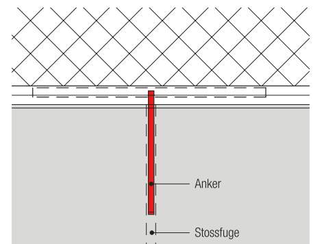
Ansicht
