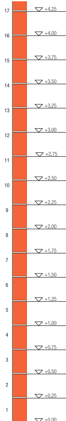
Grundform Unipor H = 238 mm
