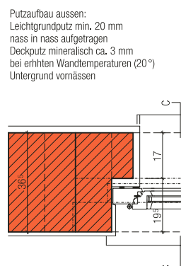
Grundriss Leibung B-B
