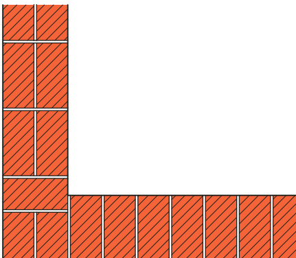
Grundriss 2. Schicht
