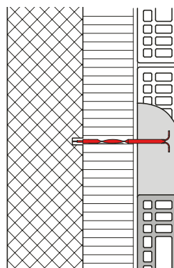
Anker bis zum Anschlag eindrehen, Anker in äussere Schale einmauern
