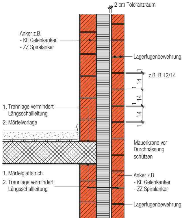
Schnitt A-A
