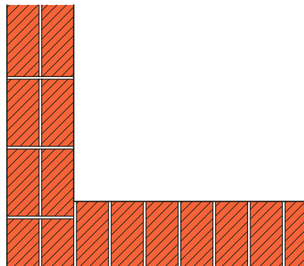
Grundriss 4. Schicht
