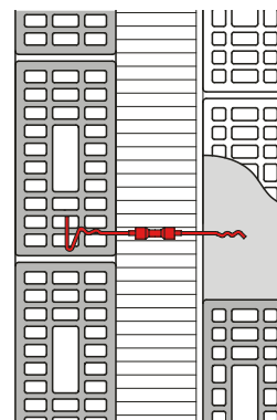
Nachziehen der äusseren Schale und Einmörteln des Ankers in der äusseren Schale
