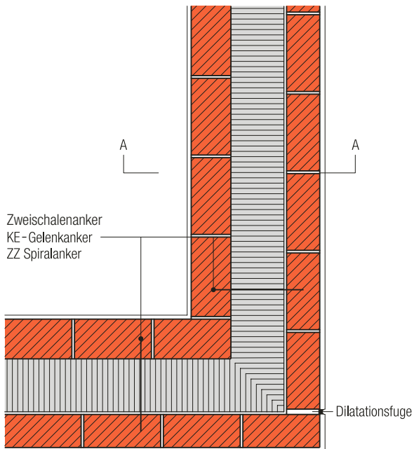
Grundriss 1. Schicht
