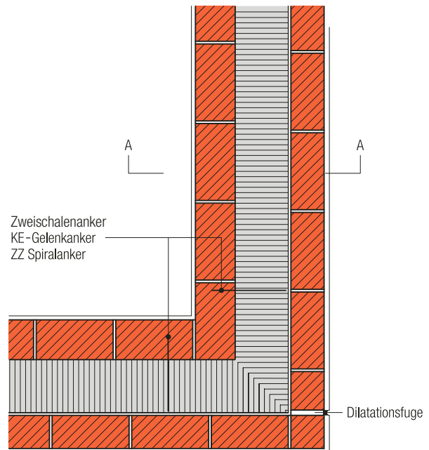
Grundriss 2. Schicht
