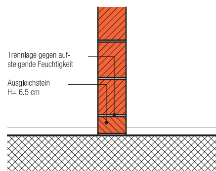
Schnitt
