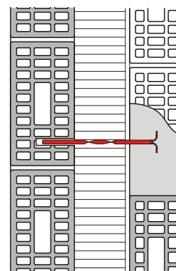
Anker bis zum Anschlag einführen, Anker in äussere Schale einmauern
