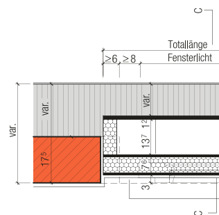
Grundriss Sturz A-A
