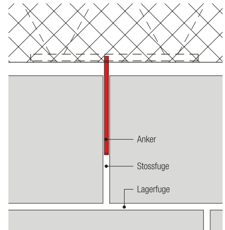
Ansicht
