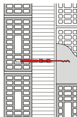
Anker bis zum Anschlag einführen, Anker in äussere Schale einmauern
